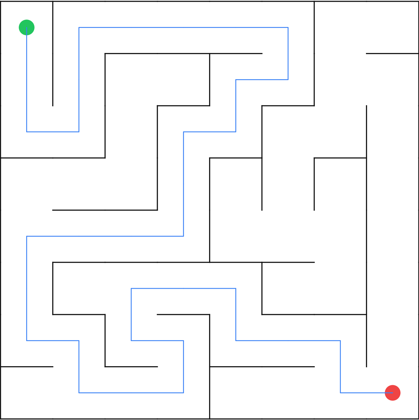
Maze 8×8 — seed 168481654
