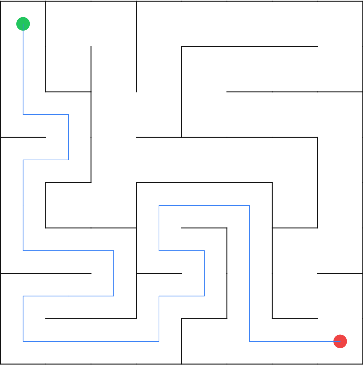
Maze 8×8 — seed 1000496071
