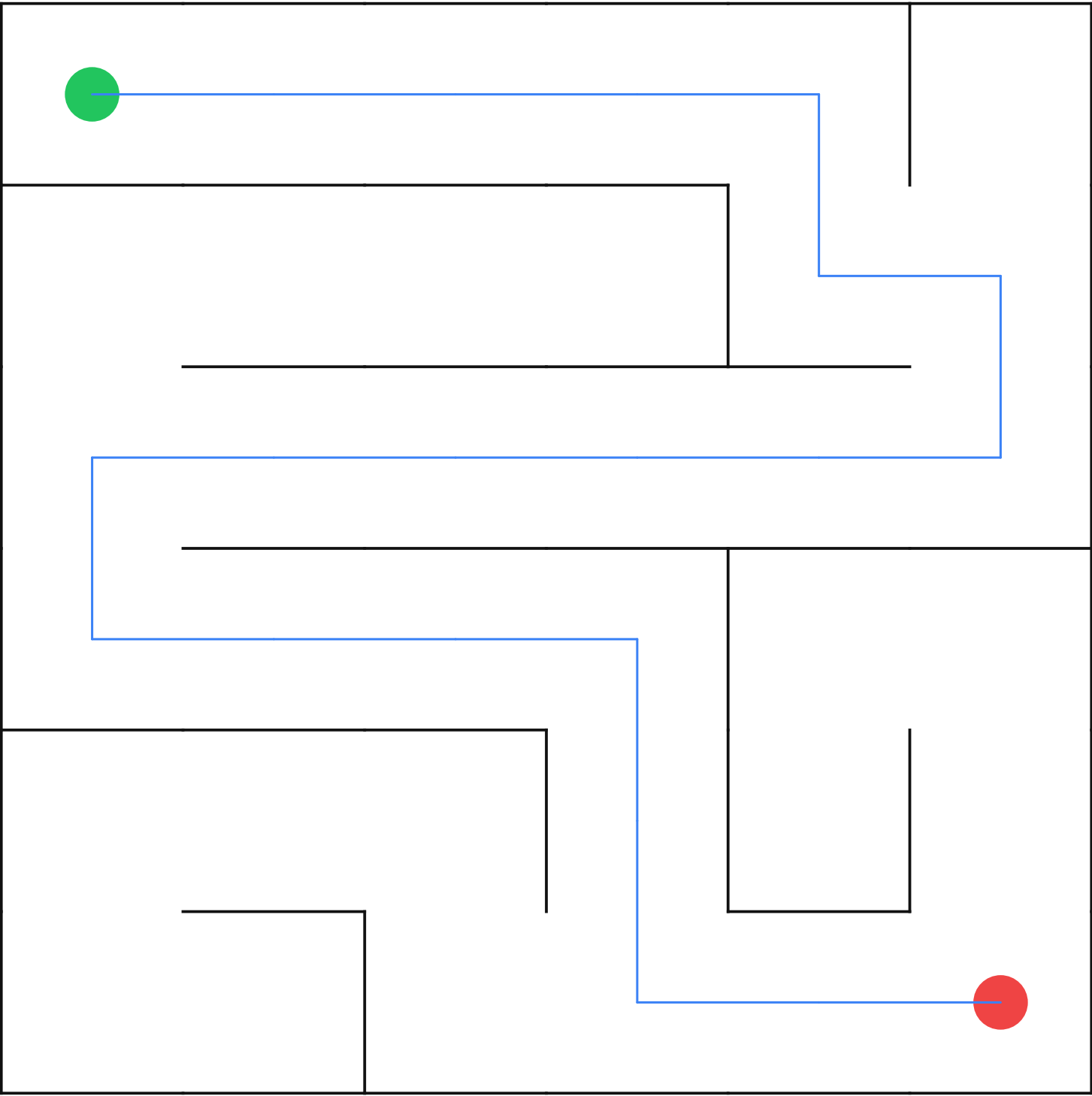
Maze 6×6 — seed 1460575758
